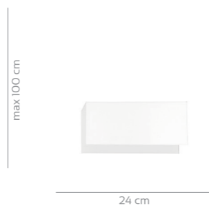
673/K1 GENTOR KI WHITE 1xE27 max 60W
